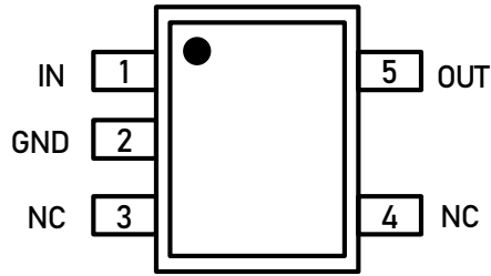
SOT23-5L
